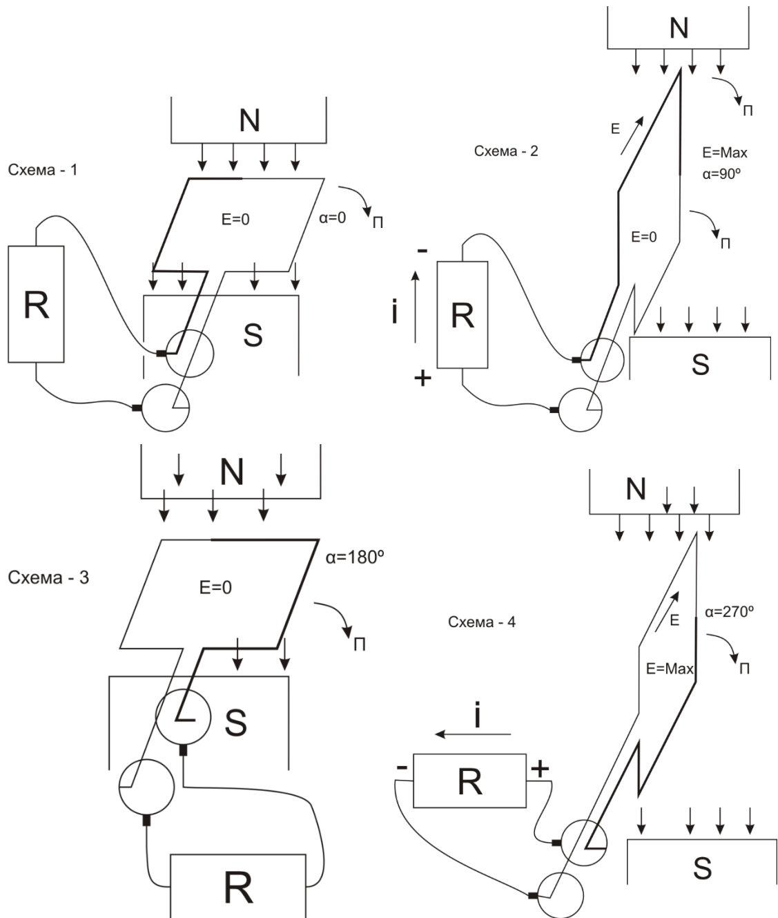
Рис.5 Вид напряжения генератора
