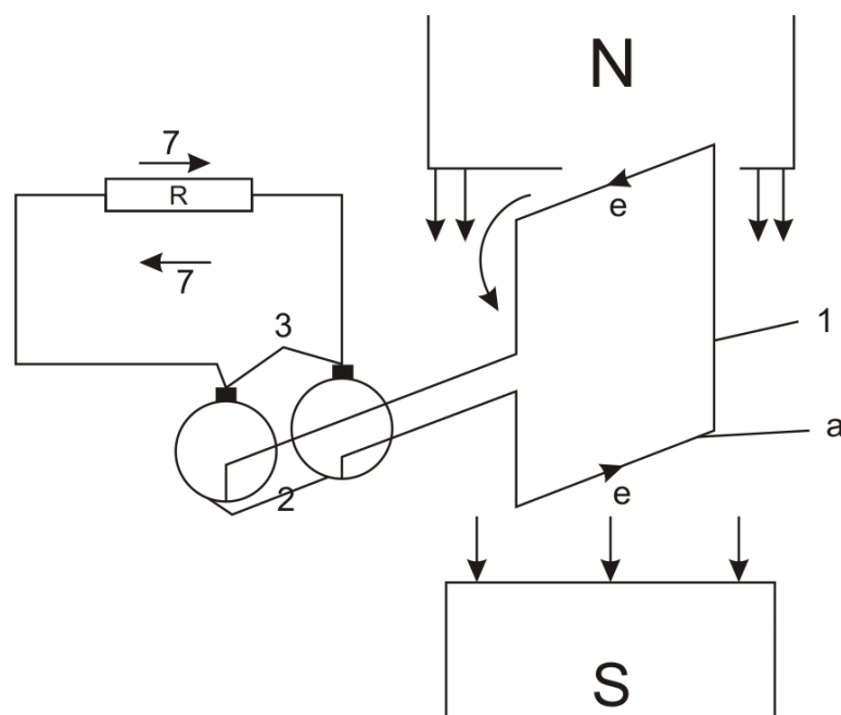
Рис.1 Схема генератора
