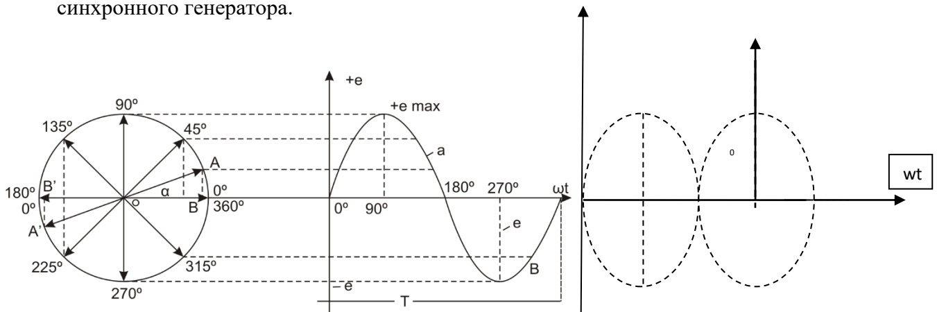
Рис.2.Временная диаграмма
